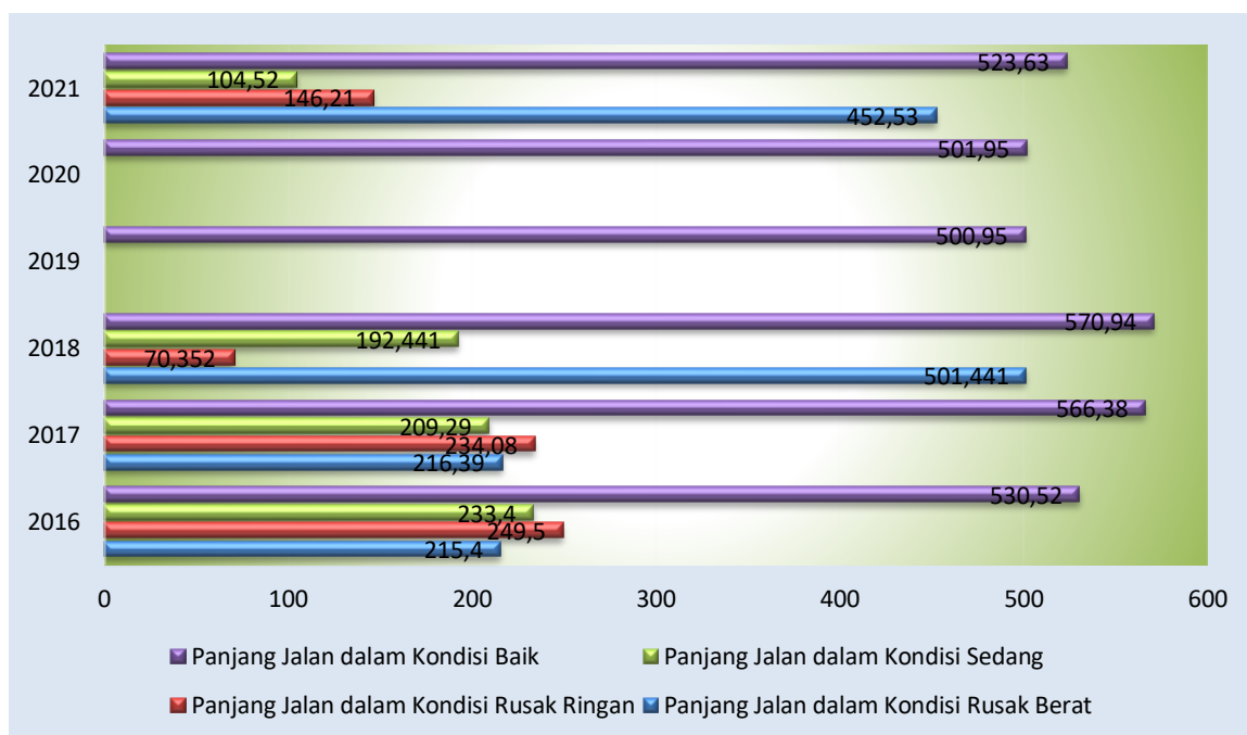
Grafik 2. 7. Panjang Jalan Berdasarkan Kondisi di Kabupaten Manggarai Barat Tahun 2016 – 2021 (Km)
