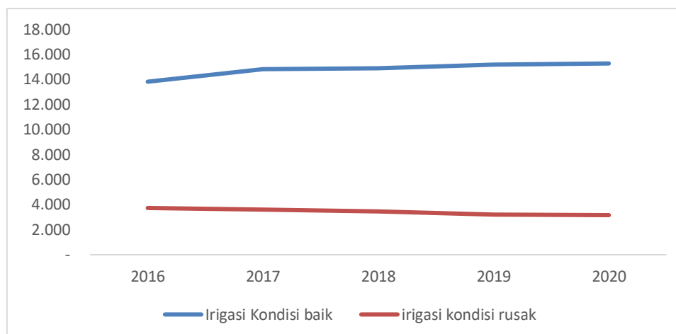
Grafik 2. 8. Proporsi Luas Irigasi dalam Kondisi Baik Terhadap Luas Irigasi Total di Kabupaten Manggarai Barat Tahun 2016 – 2020 (Ha)
